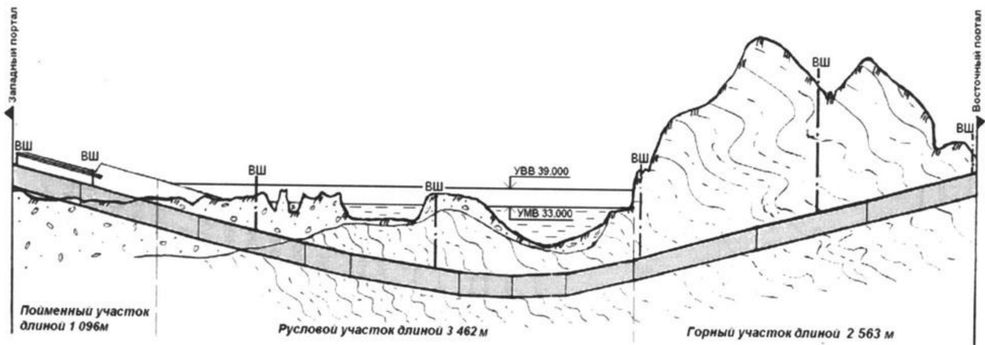
Рис. 3.1. Схема Амурского подводного тоннеля: ВШ – ось вентиляционной шахты
